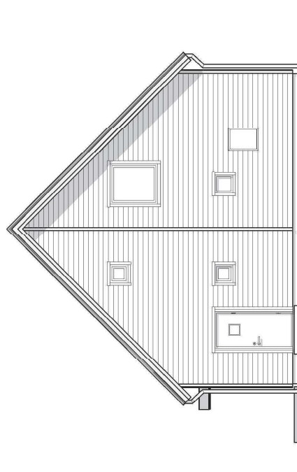
FASAD HÖGERSIDA
