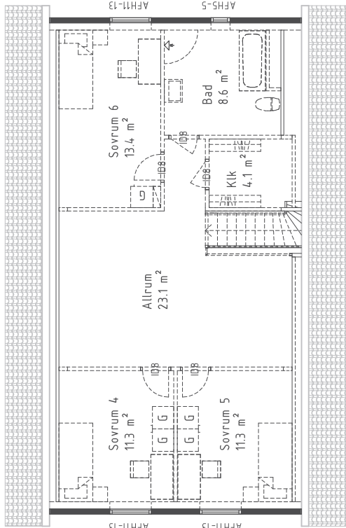
ÖVERVÅNING INREDNINGSBAR
