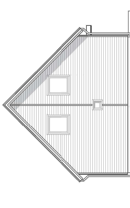
FASAD VÄNSTERSIDA
