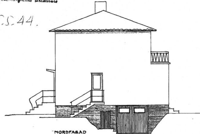
NORDFASAD
