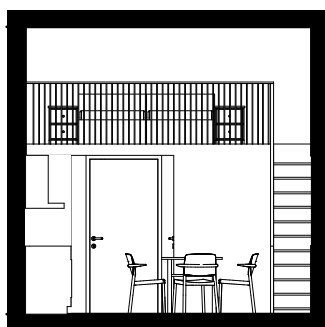
SEKTION
