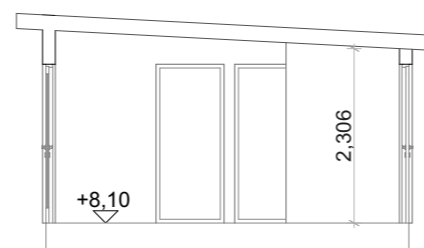
SEKTION D-D (1:100)
