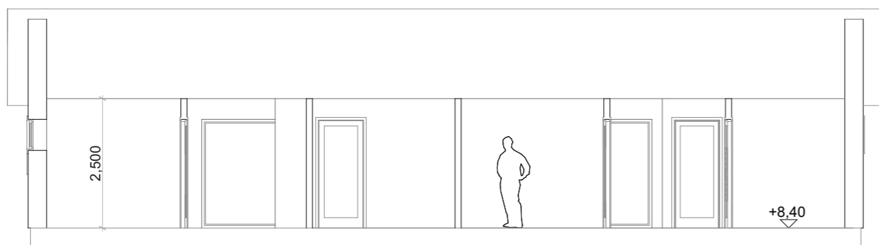
SEKTION A-A (1:100)
