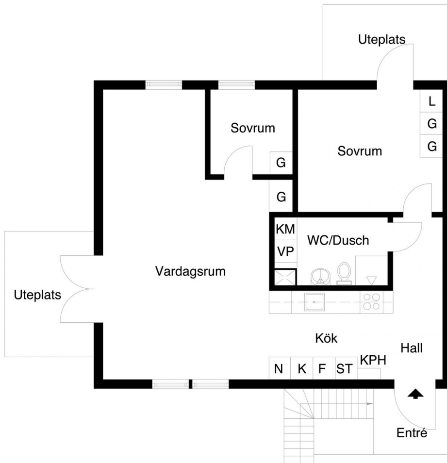
Entréplan
