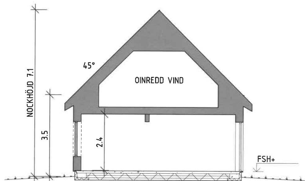
SEKTION A-A
