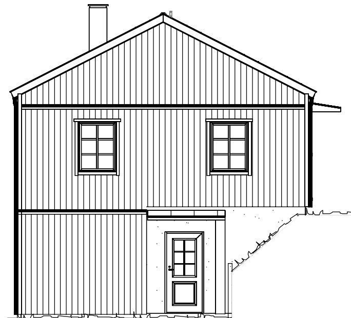
FASAD MOT NORR
