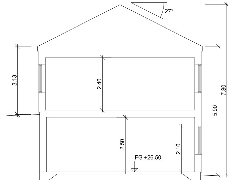
SEKTION A-A
