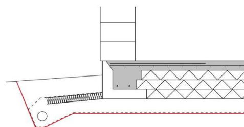
SEKTION GRUND Ovanför röd linje ingår i Dasts åtagande
