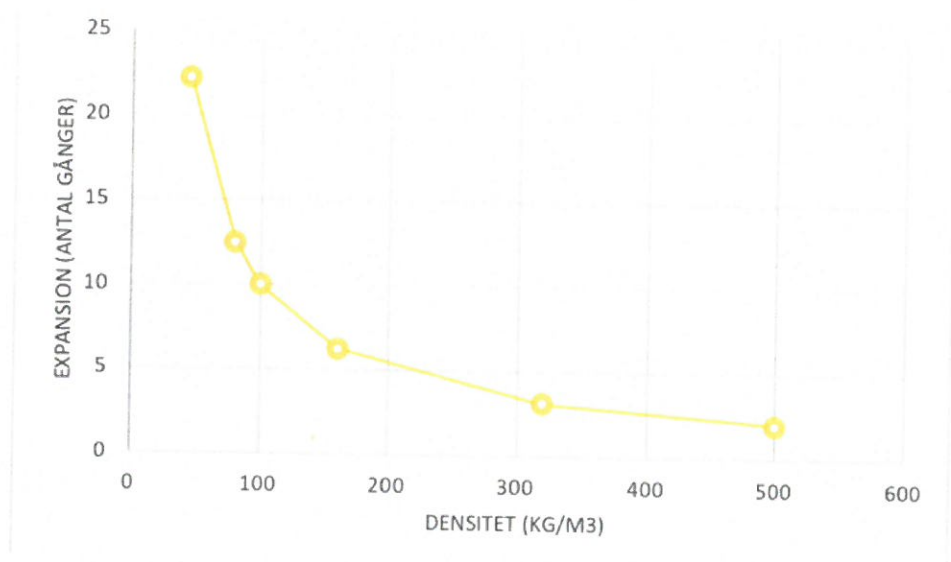
Expansionsvolym i förhållande till Stabtech® Geopolymer densiteter
