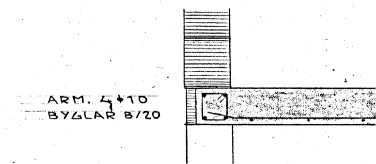
DETALJ 11 1:20
