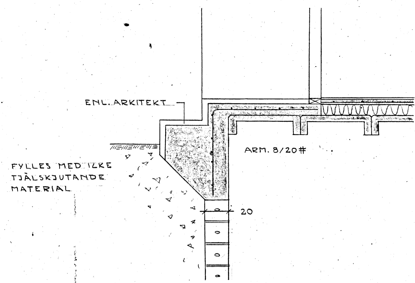
DETALJ 10 1:20
