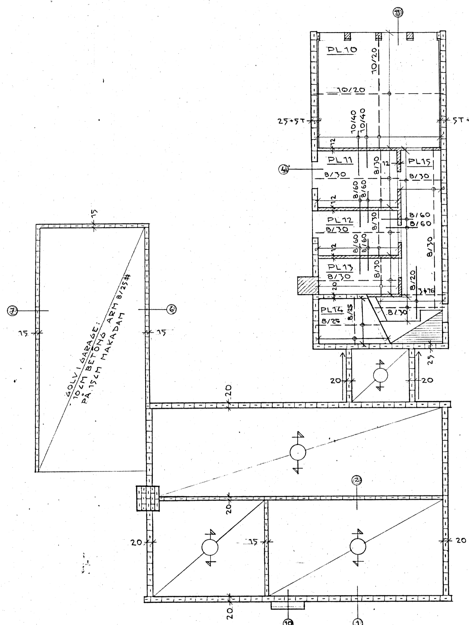
BJÄLKLAG ÖVER KÄLLAREN 1:100 PLATTJOCKLEK: PL 10 = 20CM PL 11-14 = 15CM
