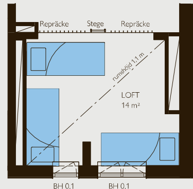
Loft
