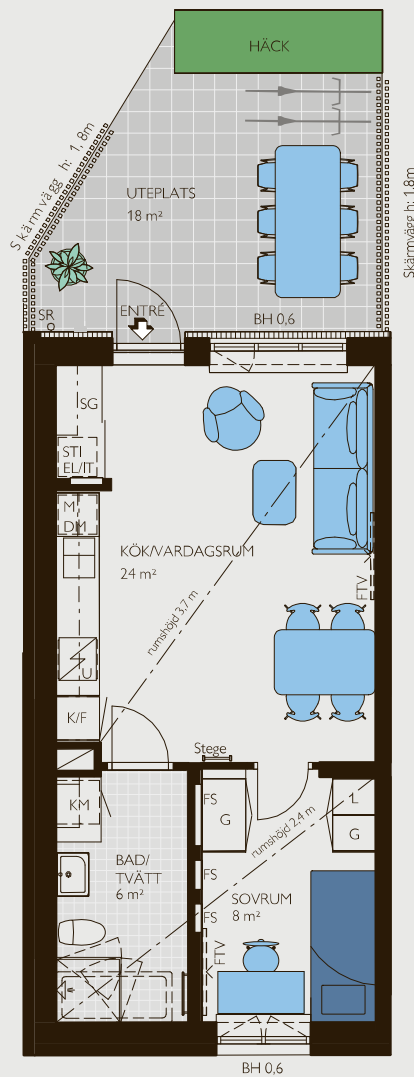
Entréplan
