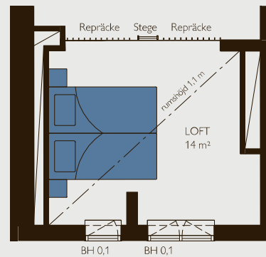
Loft
