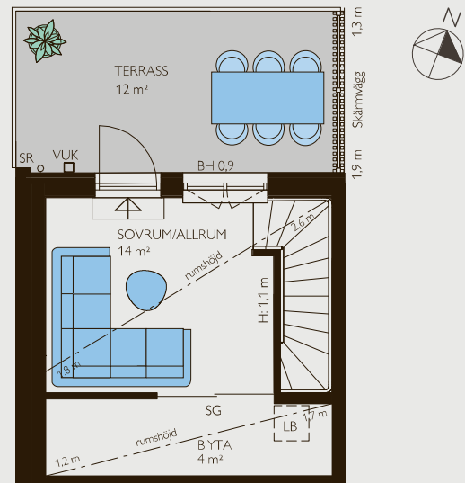
Vindsvåning
