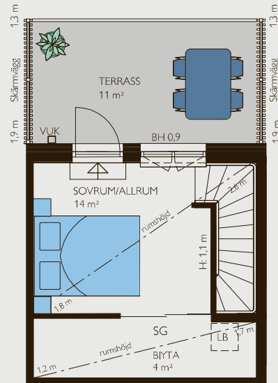
Vindsvåning
