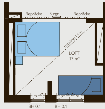
Loft
