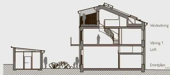
SEKTIONS RITNING
