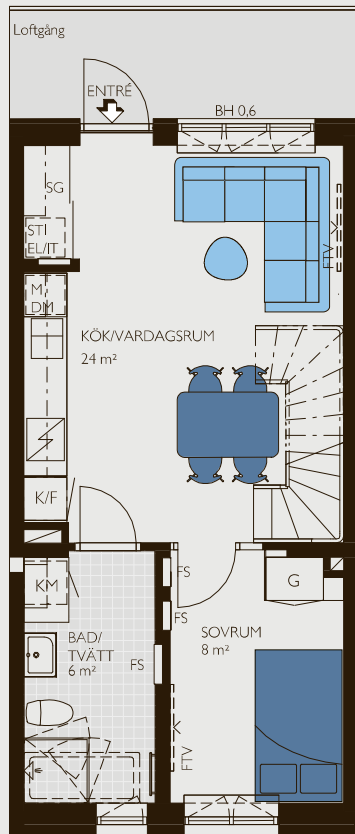
Våning 1 Rumshöjd 2,5 m
