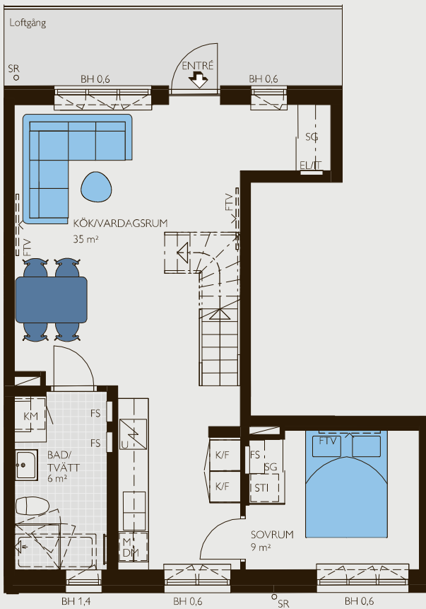
Våning 1 Rumshöjd 2,5 m
