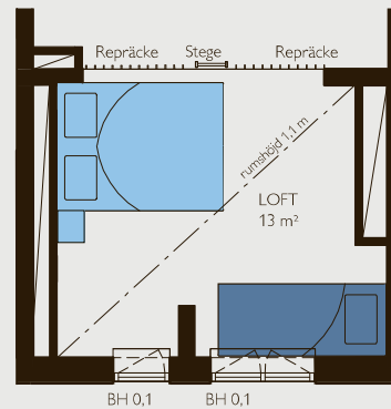
Loft
