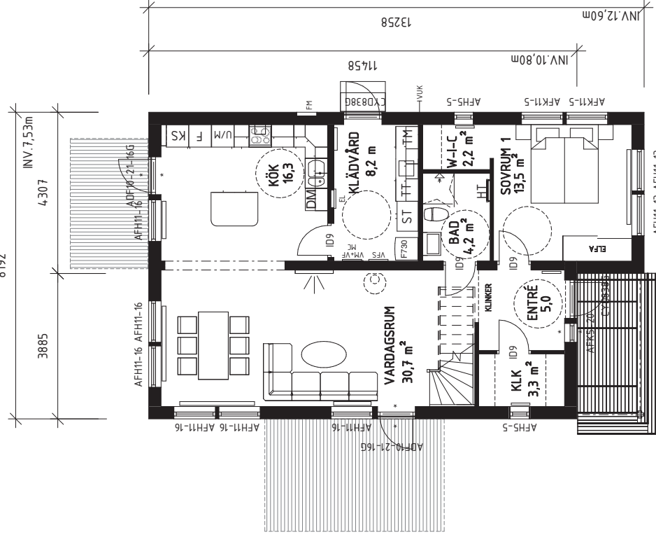
ENTRÉVÅNING
