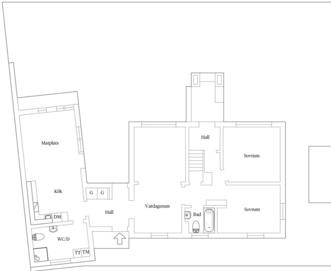
VÅNING 1
