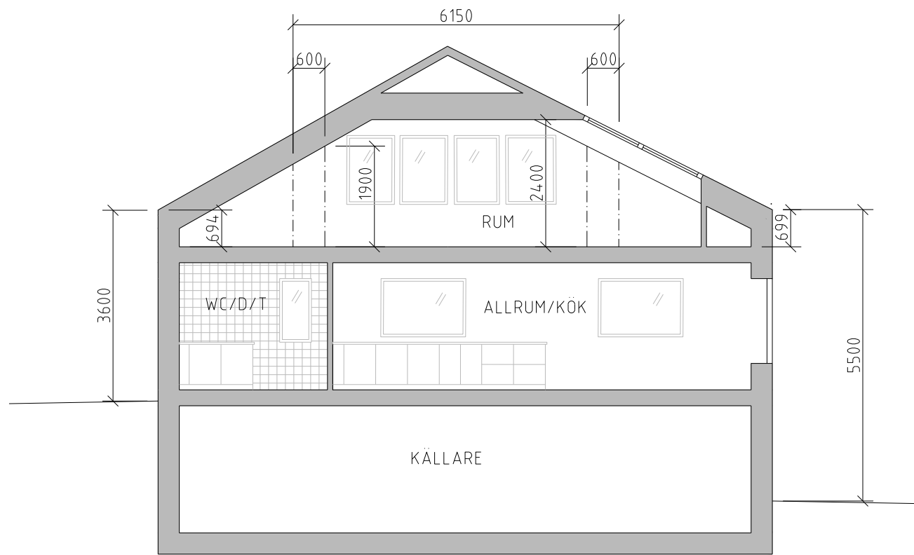
SEKTION A-A
