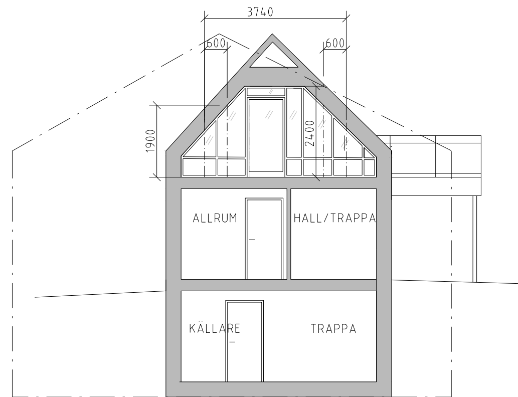
SEKTION B-B
