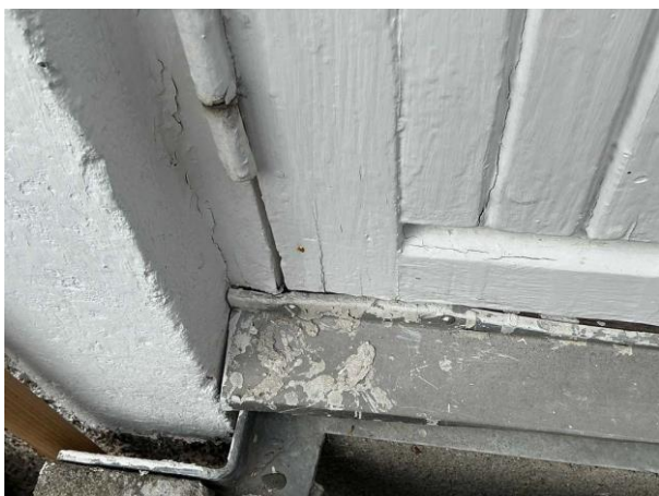
Bild 3: Utvändigt, Ytterdörr, Tröskelplåten är felmonterad samt är den inte tät mot tröskeln till dörren på baksidan
