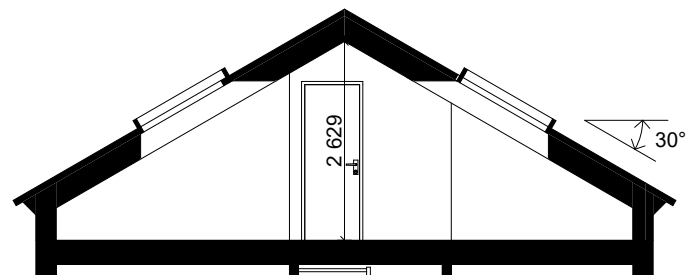
TYPSEKTION VINDSPLANET 1:100
