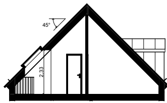
TYPSEKTION VINDSPANET 1:200
