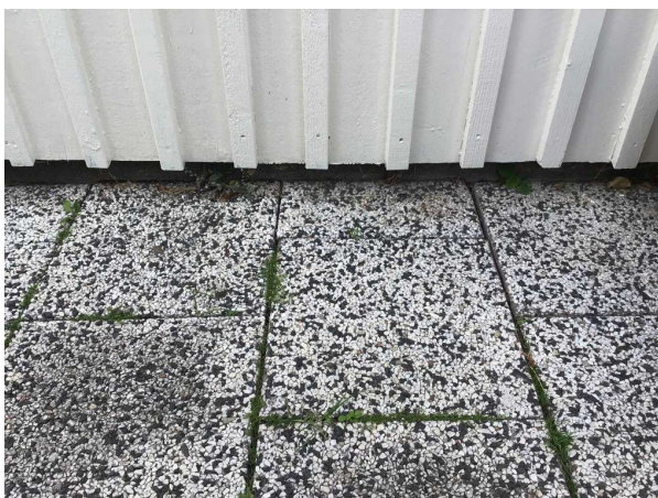
Bild 2: - Utvändigt, Fasad, Fasaden är lokalt marknära (närmare än 200 mm). Se Riskanalys.
