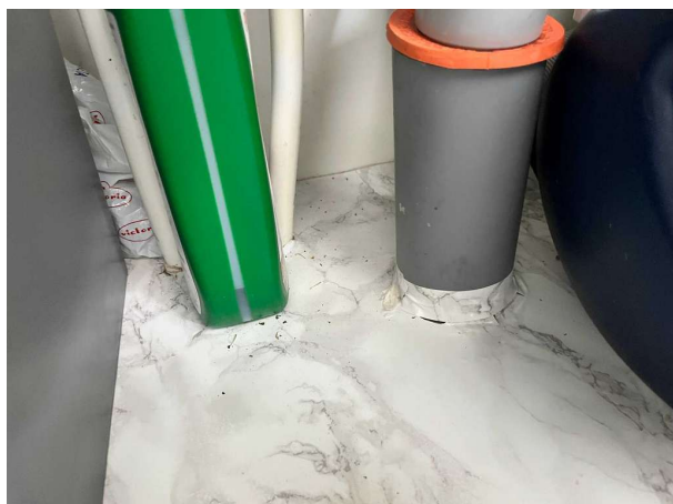
Bild 7: Invändigt, Entréplan, Bättre tätning i diskbänkskåp erfordras.
