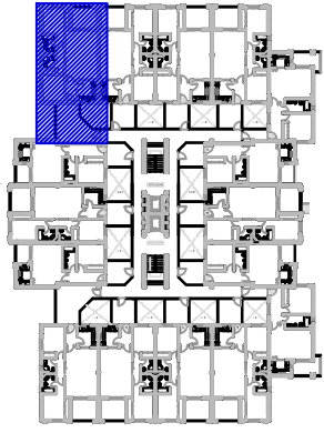
PLANTA SEGUNDA
