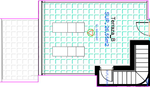
CUBIERTA ATICO_B
