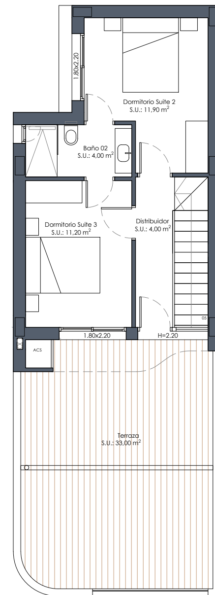
Planta primera
