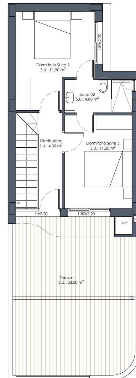
Planta primera
