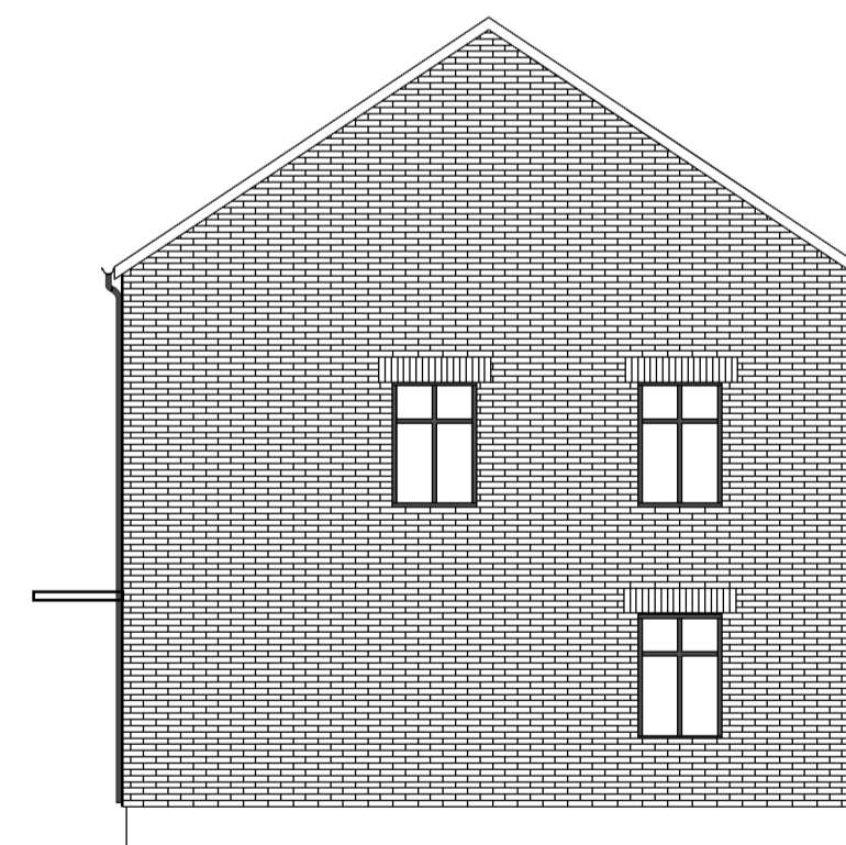
FASAD MOT PASSAGE 1 : 100
