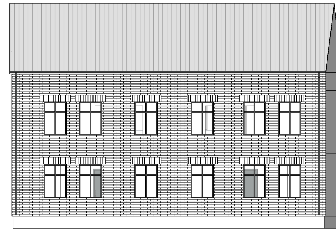
FASAD MOT RÅÅVÄGEN 1 : 100
