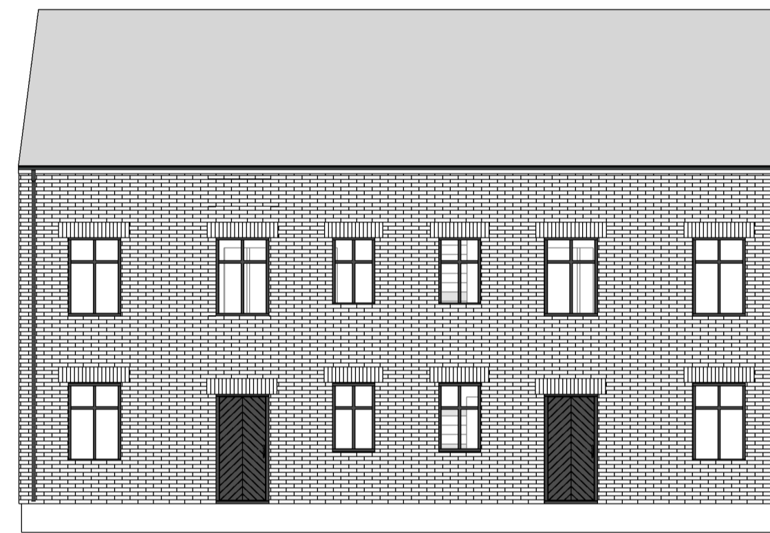
FASAD MOT GÅRD 1 : 100
