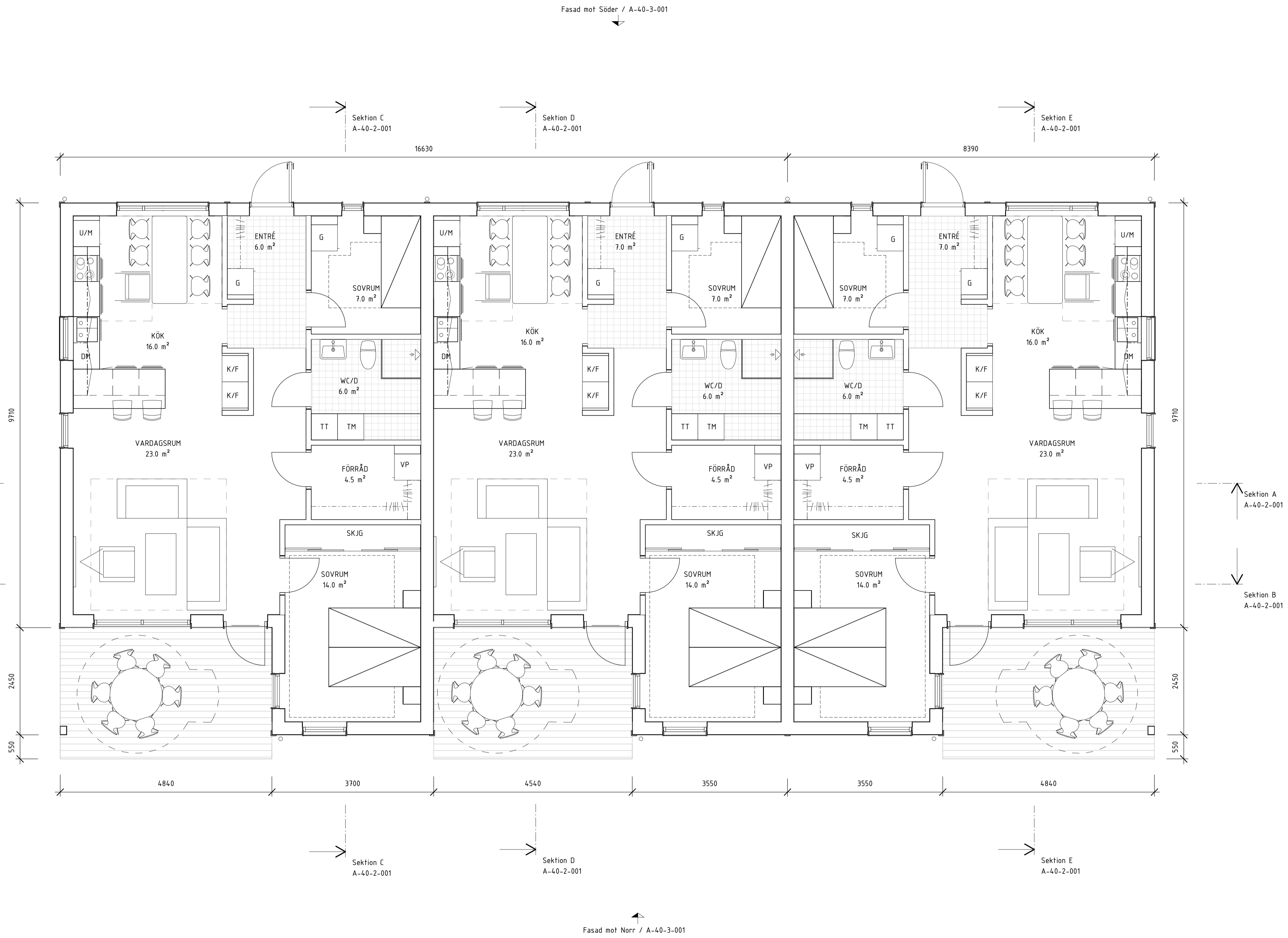
Entréplan 1 : 50
