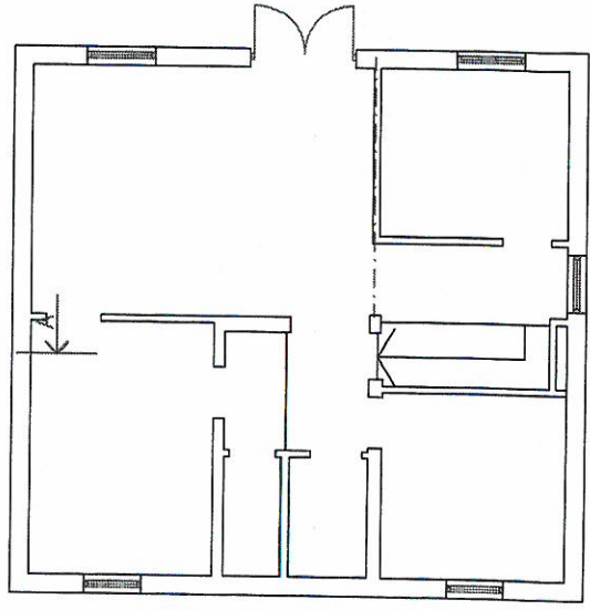
Källar plan
