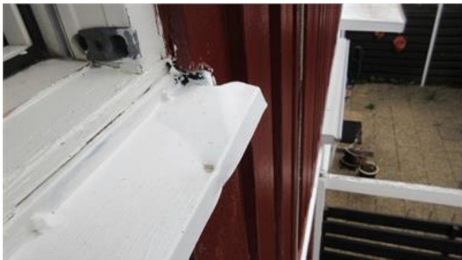
Bristfälligt/otätt fönsterbleck.
