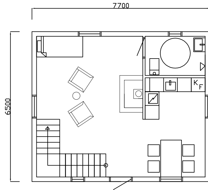
Plan 1 BOA 44,5 m 2 BYA 50 m 2
