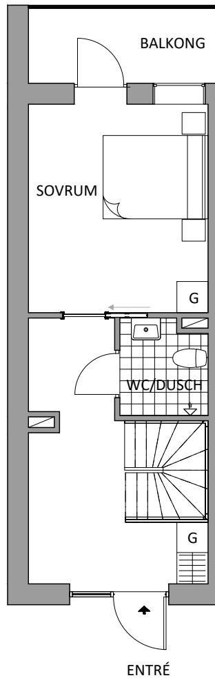
ÖVRE PLAN 32 m 2
