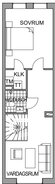
NEDRE PLAN 39 m 2
