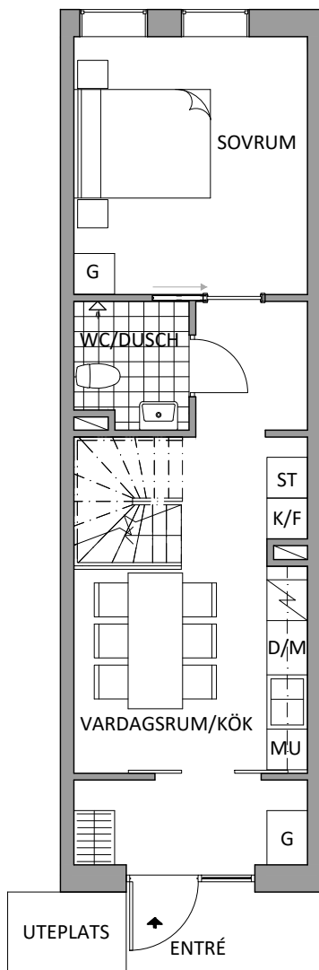
NEDRE PLAN 42 m 2
