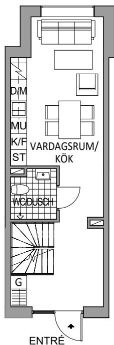
ÖVRE PLAN 36 m 2
