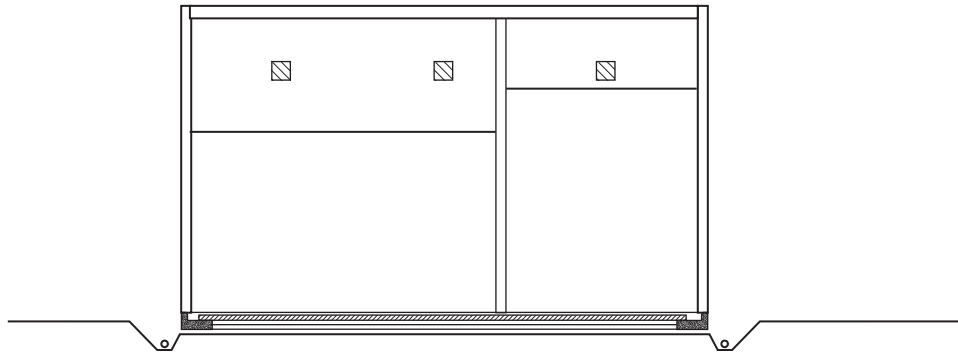
SEKTION B - B
