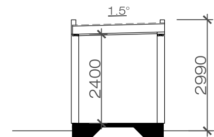
Sektion B-B
