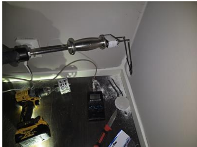
Fuktmätning sovrum 2.
