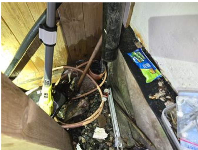
Exempel på stuprör som inte är anslutet till markrör.
