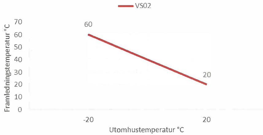
VS02 - radiatorkrets för bostäder och posten
