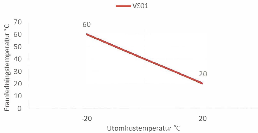
VS01 - radiatorkrets för bostäder och posten
