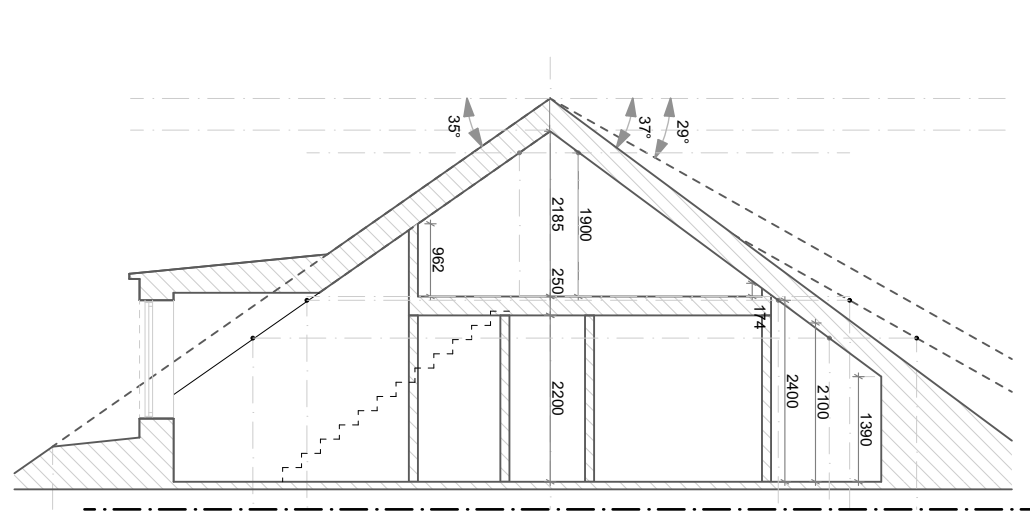
SEKTION A-A
