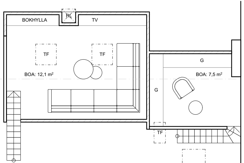
LOFTVÅNING
