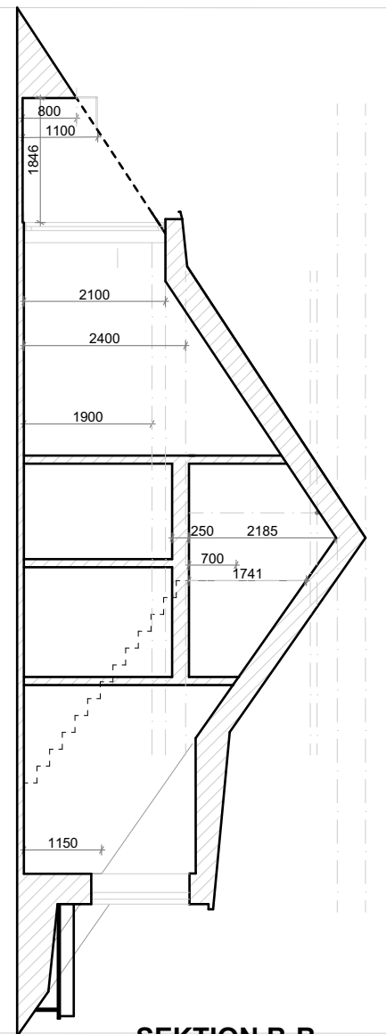
SEKTION B-B
