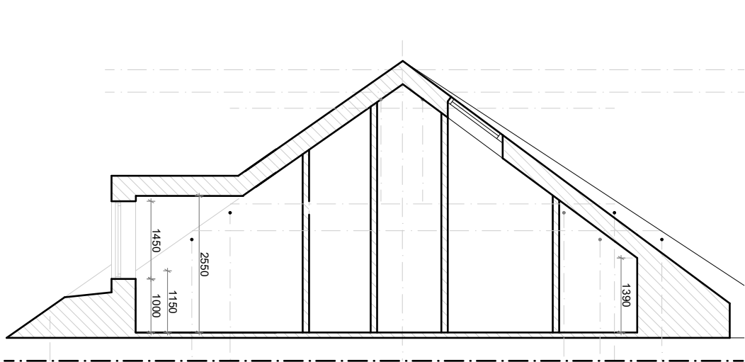
SEKTION A-A
