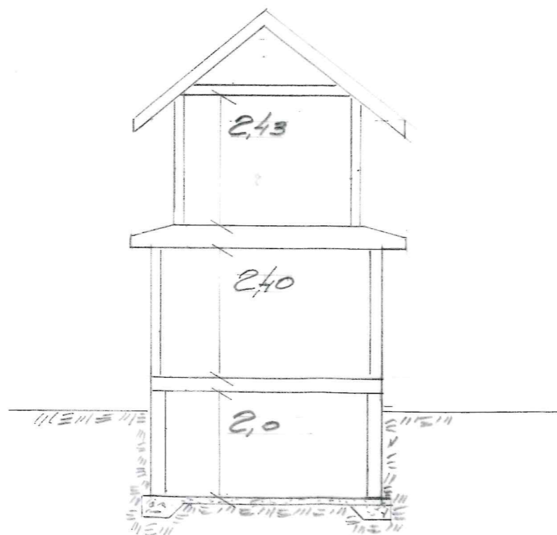
sektion tillbyggnaden
