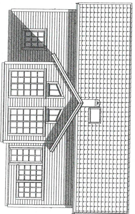
Fasad 3
