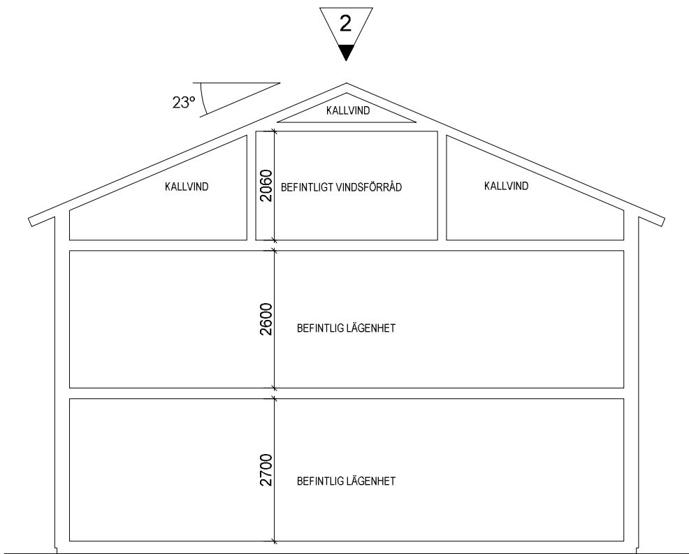
D-D BEFINTLIG DEL SOM INTE BERÖRS AV OMBYGGNADEN
