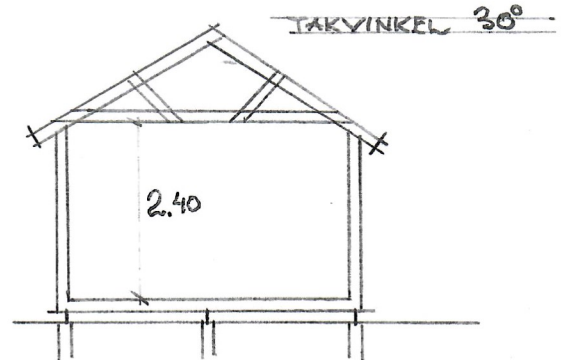
SEKTION
