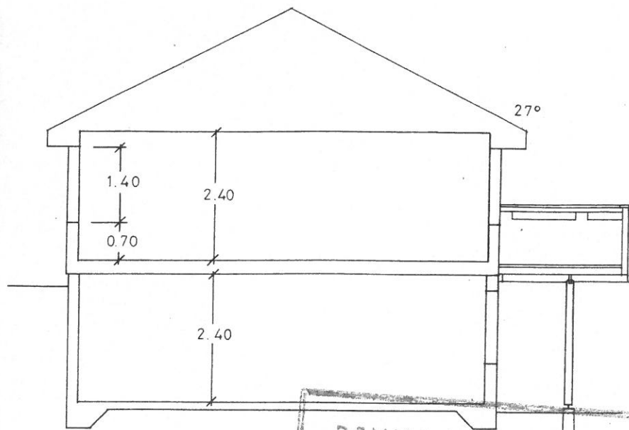
SEKTION
