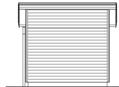
FASAD MOT VÄNSTERSIDA
