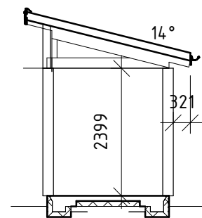
Öppen kort takfot SEKTION
