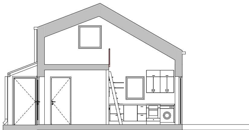
SEKTION
