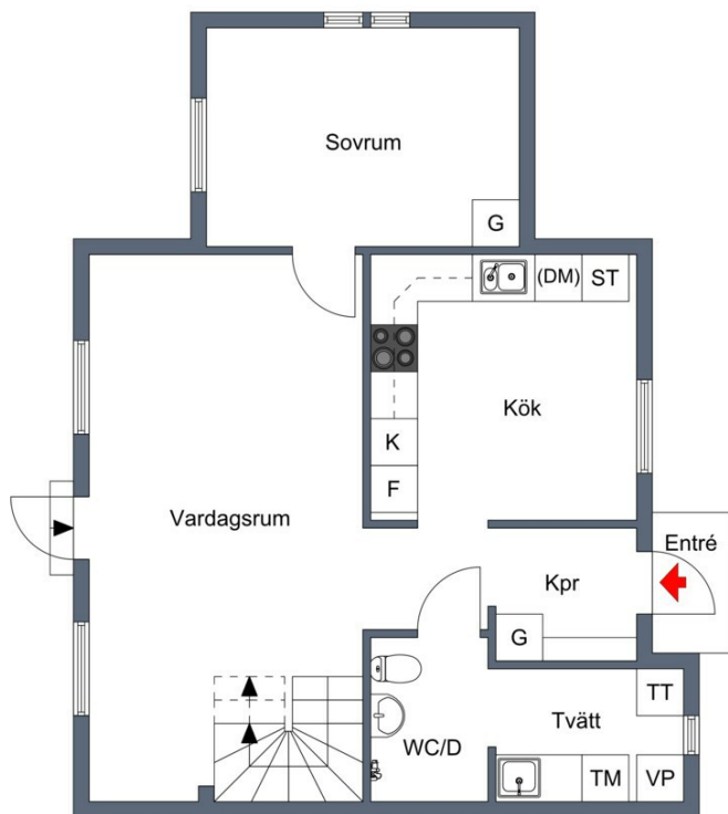
Planskiss entréplan
